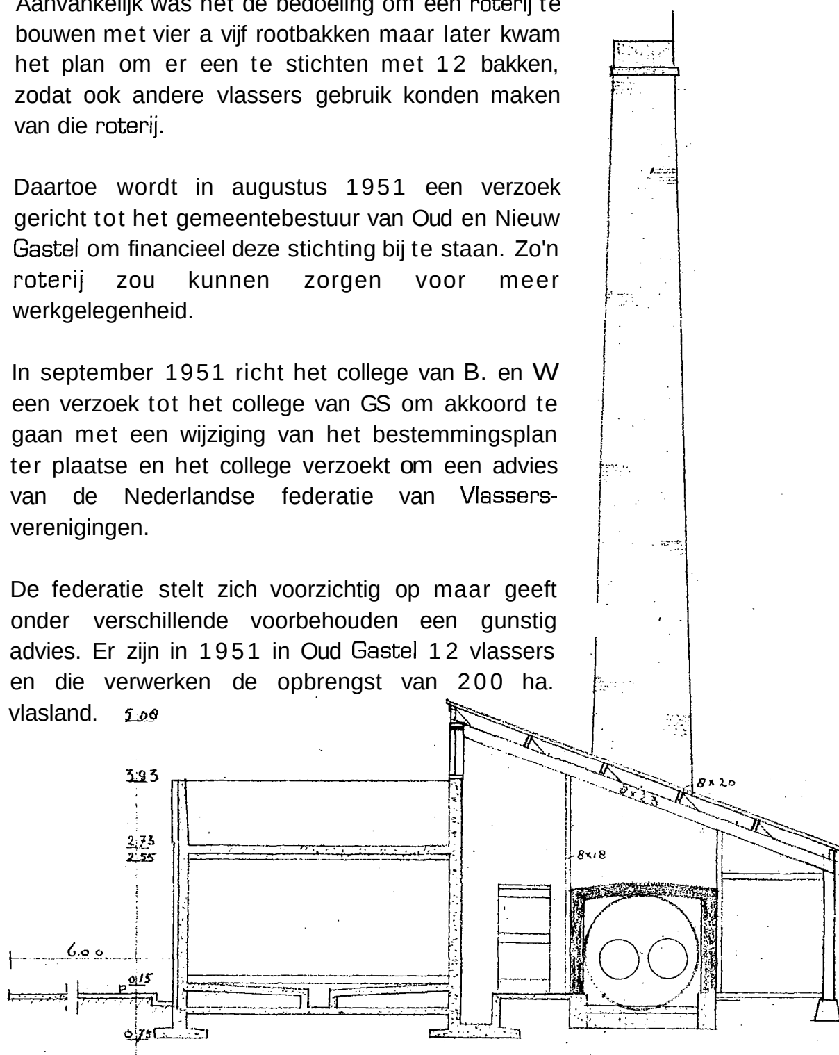
DOORSNED E A-B
