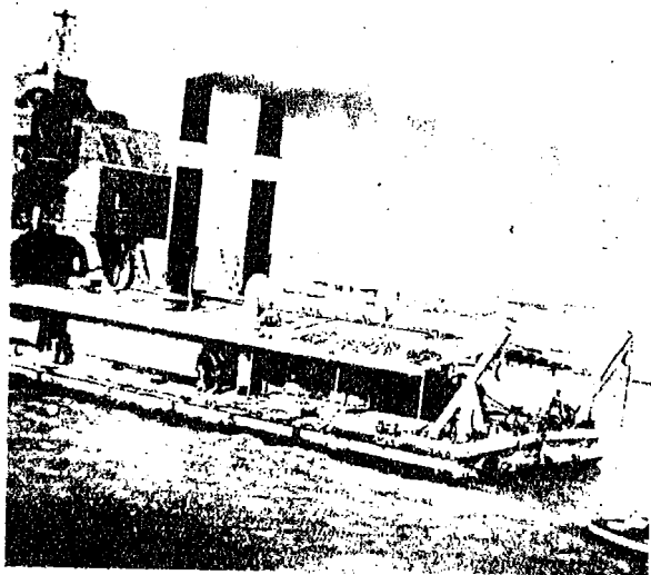
NEDERLANDSE BAGGERMOLEN aan het werk in het Suezkanaal.
