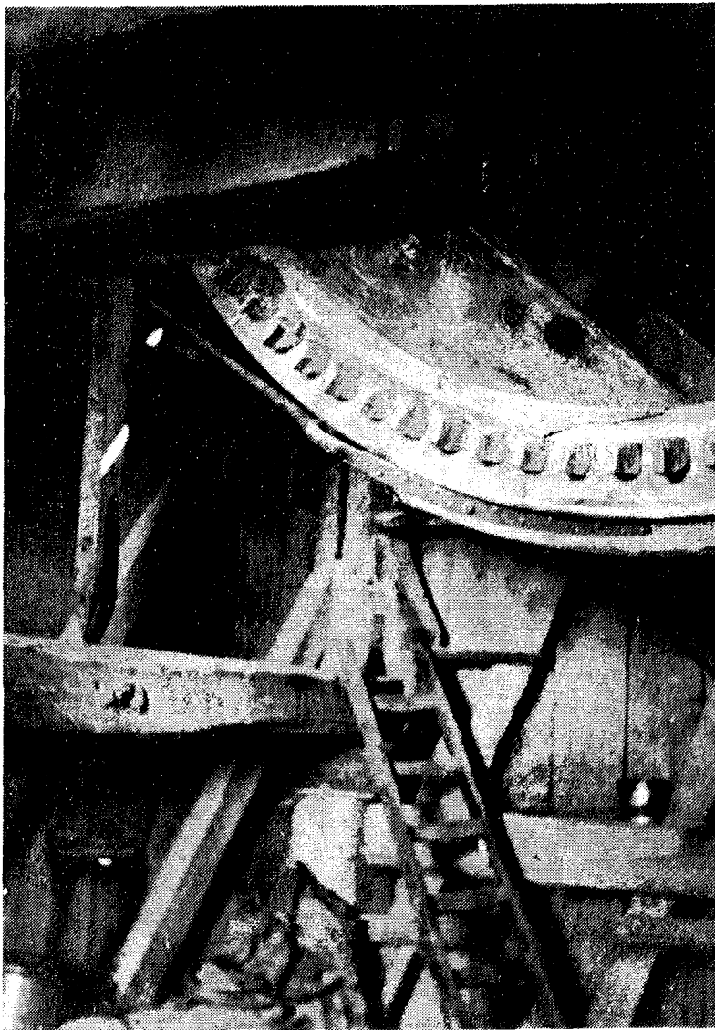
Een interieurfoto van de molen van J. Peeters. Duidelijk is het bovenwiel te zien, dat aan de wiekenas zat. Aan de onderzijde van het wiel is een gedeelte van de vang (rem) zichtbaar.
